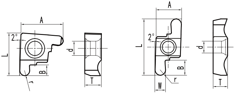
A、B 系列刀片式样 A/B Series Insert Type
